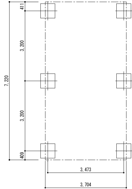
■基礎配置図
